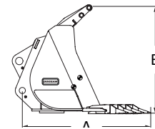
Pin-On
